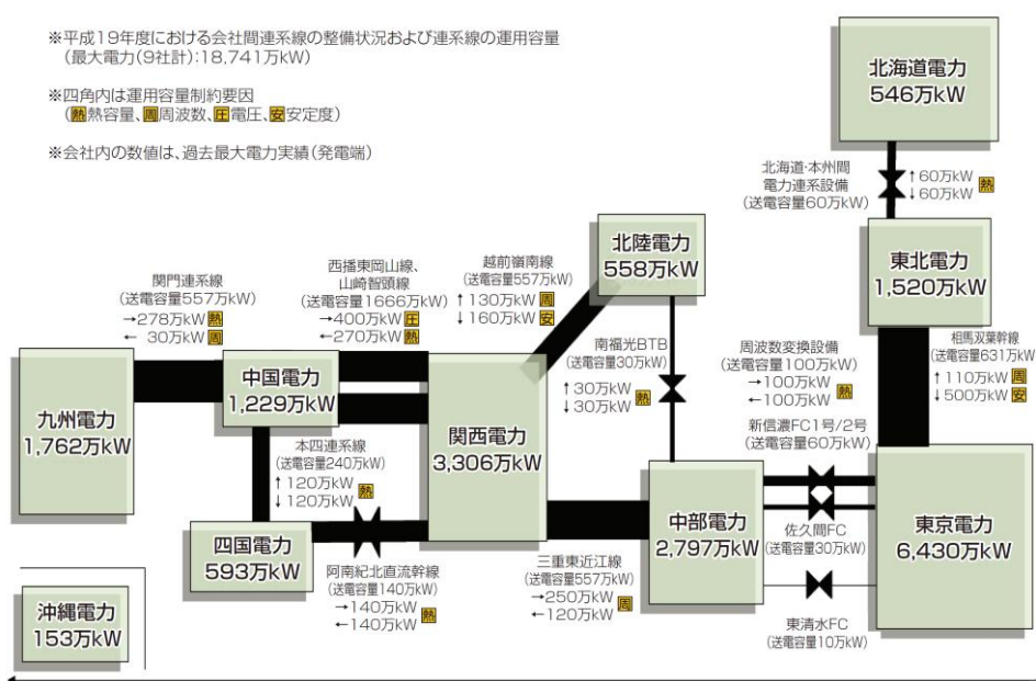
【第111-2-7】連系線と運用容量
