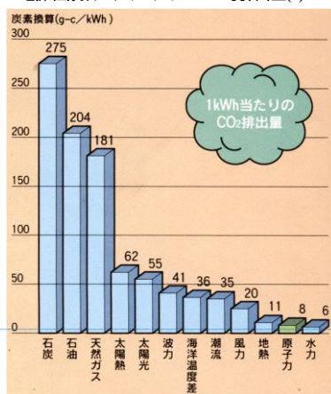
電源種類別のライフサイクルCO 2 排出量(1)
