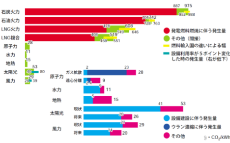
ライフサイクルCO 2 の排出量 (メタンも考慮)
