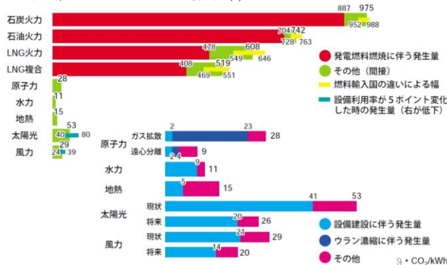
電源種類別のライフサイクルCO 2 排出量(2)
