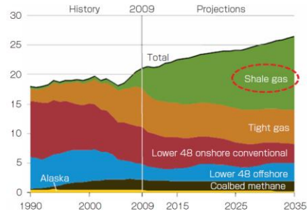
【第 121-4-2】米国の天然ガス生産推移・見通し(種類別)
