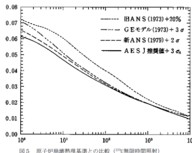
図5 原子炉崩壊熱現基準との比較 (2011無限時間照射)
